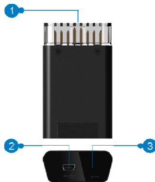
Fig. 1-2 VCI module
