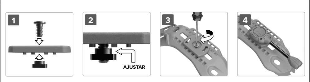
Figura 7 – Instalación con montaje MICH
