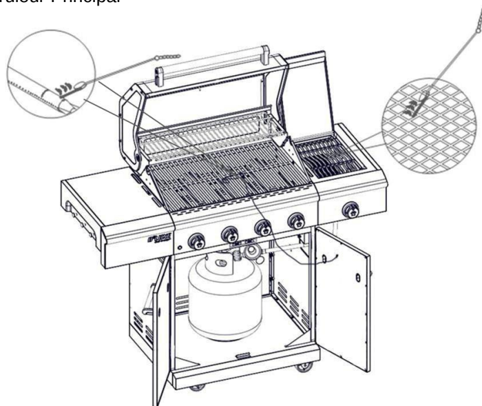
Brûleur Principal
