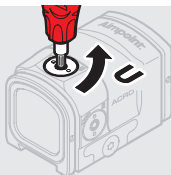
Fig. 4 Réglages en site
