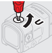
Fig. 4 Ajustes de elevación
