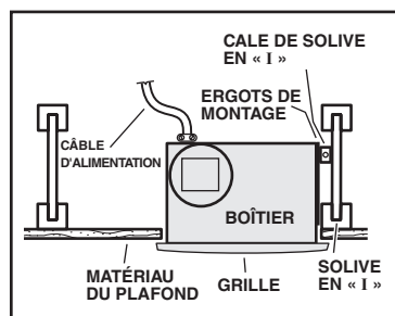
Boîtier fixé aux solives en « I ».
