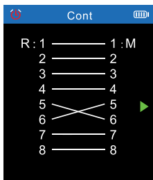
Kabelkreuz
