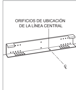
Soporte antivuelco
