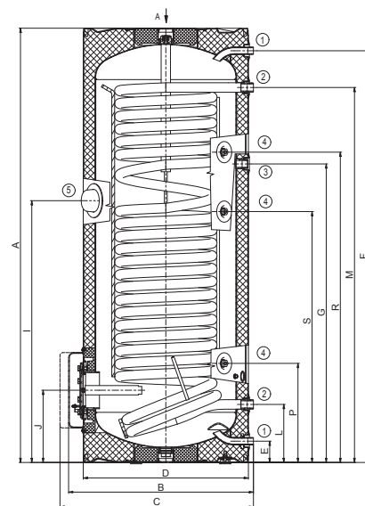
OKC 250 NTR/HP
