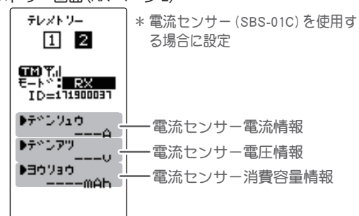
テレメトリー画面 (RX ページ 2)
