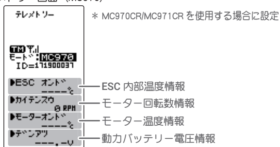
テレメトリー画面 (MC970)
