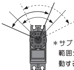
サーボホーンのセンター位置を調整
