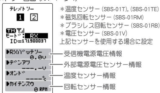
テレメトリー画面 (RX ページ 1)
