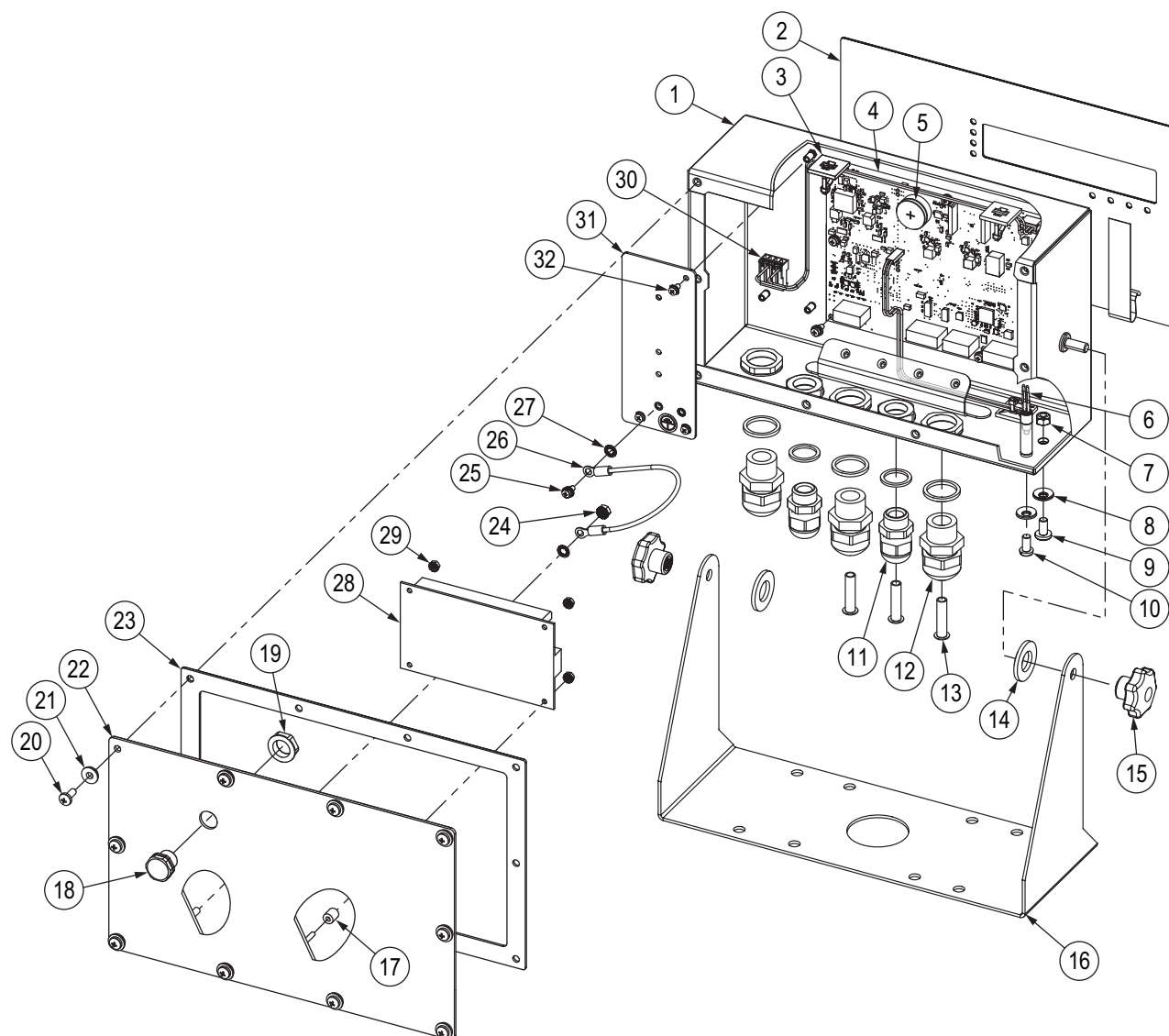
Figura 2-15. Diagrama de repuestos de modelos 680 de CC
