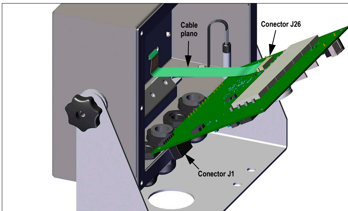
Figura 10-2. Instalación de la tarjeta de reemplazo
