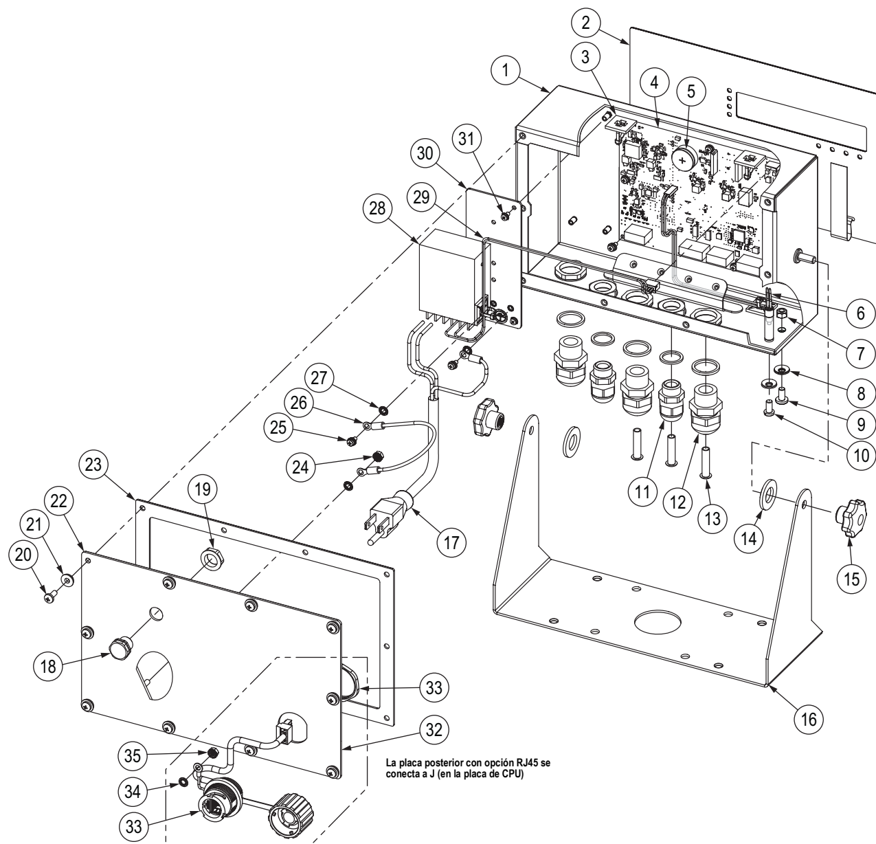
Figura 2-14. Diagrama de repuestos de modelos 680 de CA
