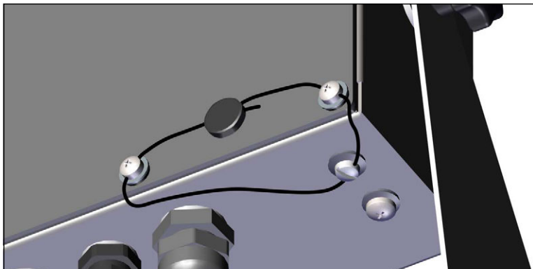
Figura 2-13. Precintado del indicador, prevención del acceso
