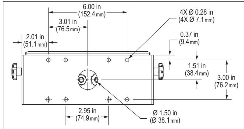
Figura 2-2. Medidas de montaje
