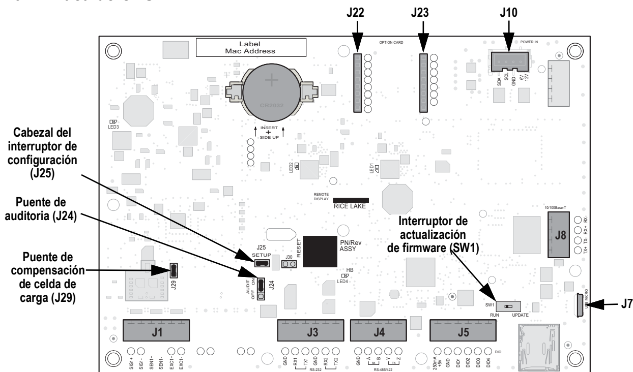
Figura 2-11. Tarjeta de la CPU 680
