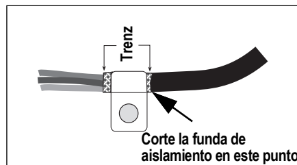
Figura 2-7. Cable con blindaje trenzado
