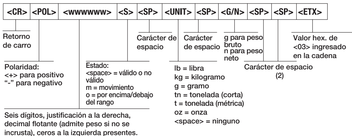
Figura 11-2. Formato de transmisión de datos Cardinal
