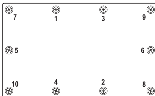
Figura 2-12. Secuencia de apriete de placa posterior
