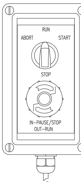
Figura 9-1. Interruptor de dosificación
