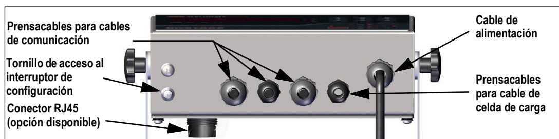
Figura 2-5. Ubicaciones recomendadas para los prensacables
