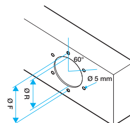
Diffuseur AR 190 - Montage sur gaine rectangulaire
