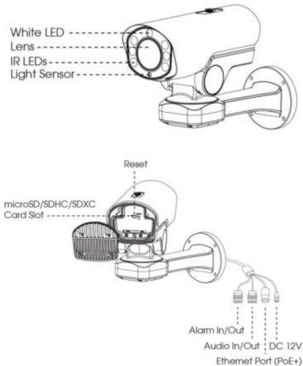
Figure 1-3-3 AI 5X/20X/23X Mini PTZ Bullet Plus Network Camera
