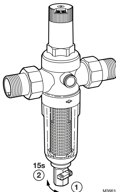
Fig. 3. Rinçage du filtre.
