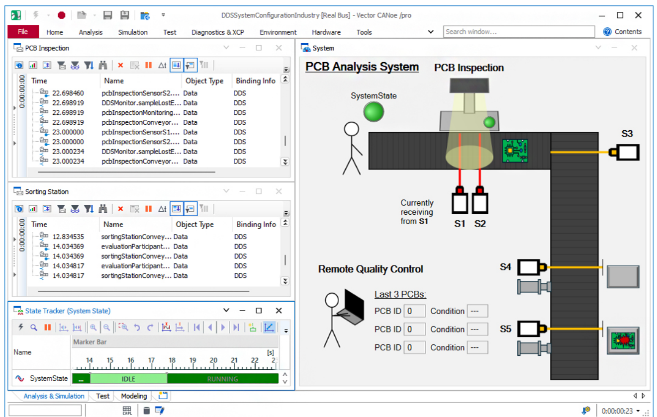
図 2: CANoe での DDS システムのシミュレーションと視覚化
