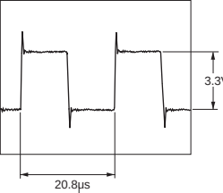
(WF06) DIGSDO (SD-9:D4)
