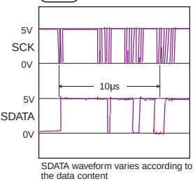
(WF61) SD-13:D2, F2
