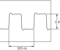
(WF08) DIGCLK (SD-9:D4)
