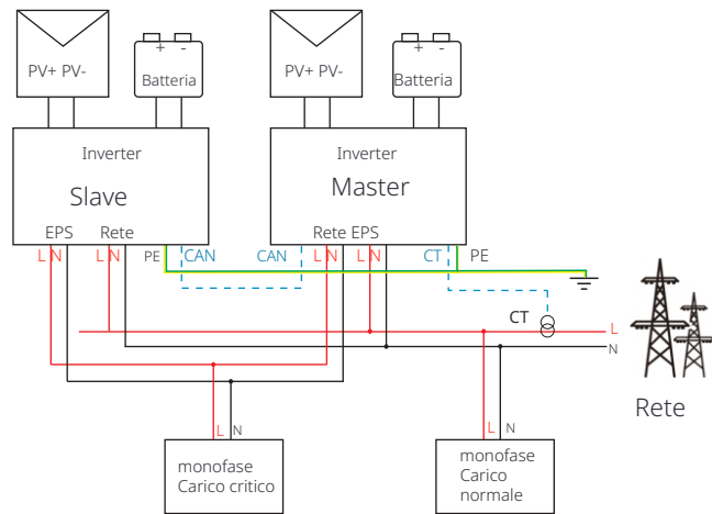
Schema del sistema applicato al sensore di temperatura CT:
