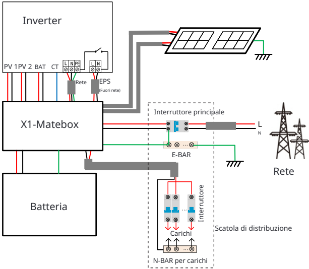
Diagramma D: La linea neutra e la linea PE sono combinate insieme, tutti i carichi si collegano alla porta EPS (fuori rete); (Applicabile all'Australia)
