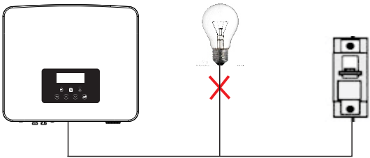
Figura: Collegamento errato del carico e dell'inverter
