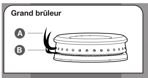
A Flamme supérieure (principal) B Débit thermique minimum (flamme de mijotage)
