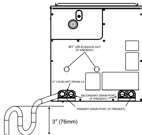
Fig. 8 – Condensate Trap
