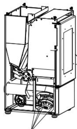
Desconecte o fio do ventilador de exaustão de fumaça e use uma chave Allen de 4 mm para desenroscar o parafuso de fixação e removê-lo para limpeza
