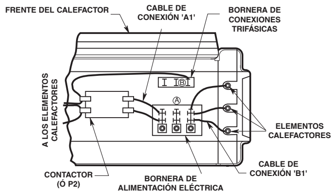
CABLEADO EN FÁBRICA PARA ALIMENTACIÓN MONOFÁSICA
