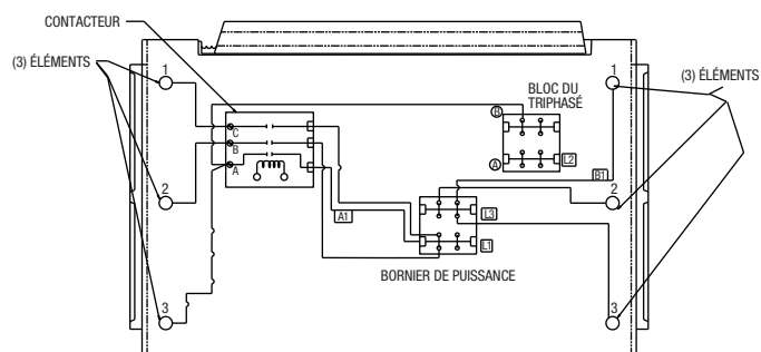
CÂBLAGE D'USINE POUR ALIMENTATION EN MONIPHASÉ
