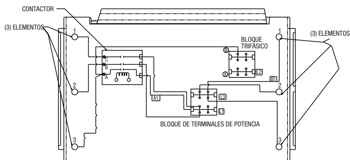
CABLEADO EN FÁBRICA PARA ALIMENTACIÓN MONOFÁSICA
