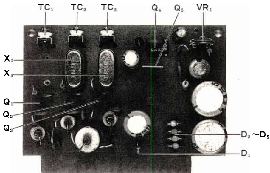
Fig. 17 REG-BFO UNIT
