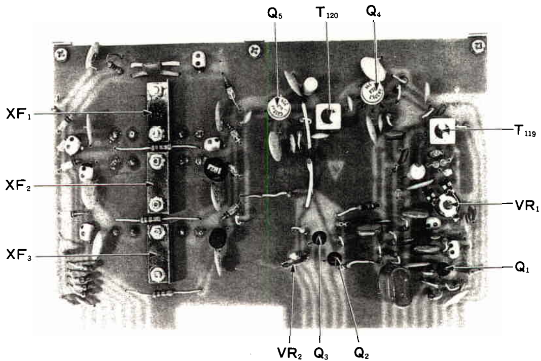
Fig. 15 IF UNIT
