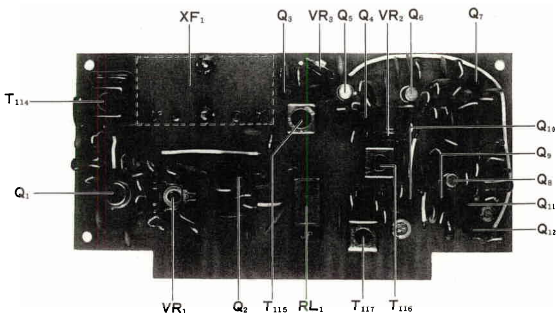
Fig. 14 NB-MIX UNIT
