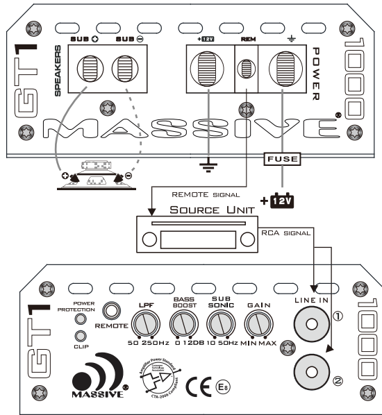
FIG 4. MONO AMOLIFIER WIRING GT 1
