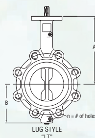
LUG STYLE "LT"
