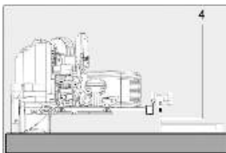
Fig. 34: Colocar la máquina sobre el riel guía
