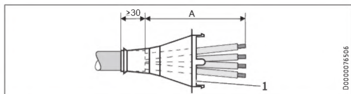
1 Kabeltulle
