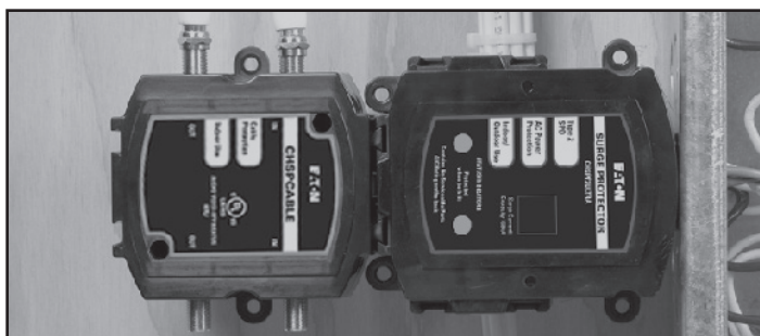
Figure 7. Joining CHSP Modules (1)/Jonction de modules CHSP (1)/Conexión de los módulos CHSP (1)
