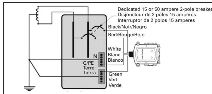
Figure 6. Wiring the CHSPT2SURGE/ULTRA/Câblage du CHSPT2SURGE/ULTRA/Conexión del CHSPT2SURGE/ULTRA
