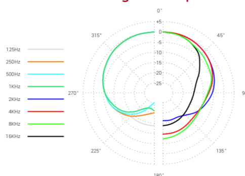
Diagramma polare
