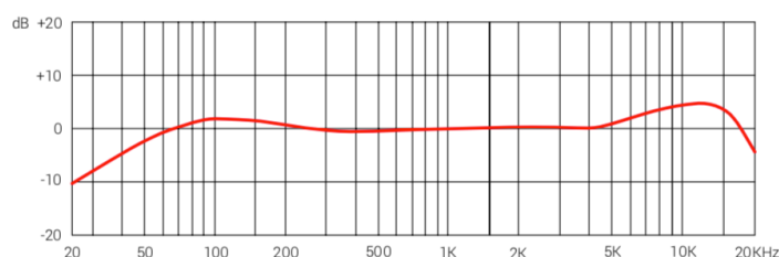
频率响应
