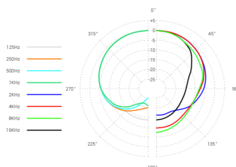
指向性
