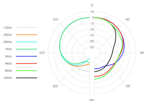
Диаграмма направленности
