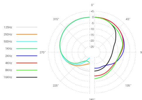
Patrón polar
