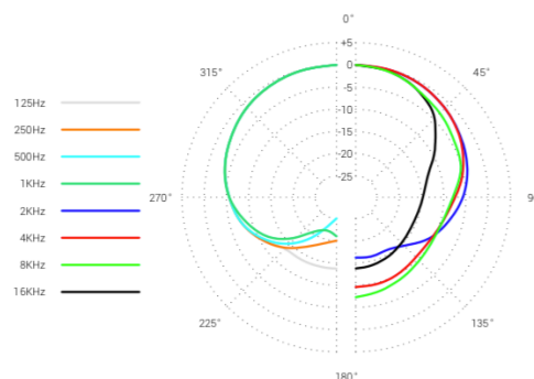
Modèle polaire
