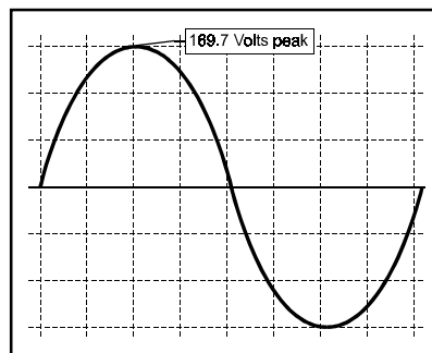
Figure 6. Onde sinusoïdale en sortie du convertisseur Sine Wave (modèle 120V AC)
