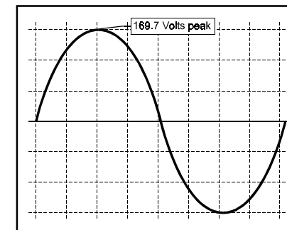
Figura 6. Salida Sinusoidal Real del Inversor Sine Wave (Modelo de 120V de CC)
