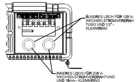
Abb. 3. Anschlußklemmen des Sine Wave-Wechselrichters für die Wechselstromverdrahtung (nur bei festverdrahteten Modell-Versionen)
