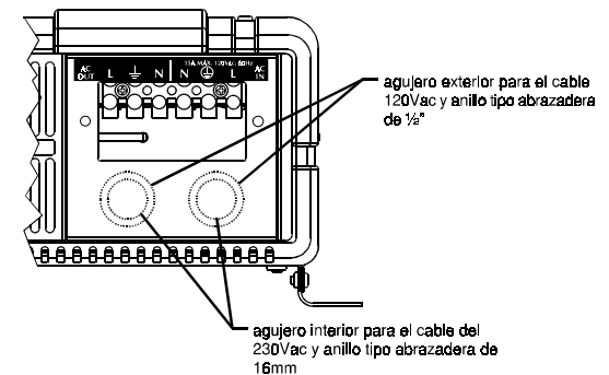
Figura 3. Terminales del Cable de CA del Inversor Sine Wave (solo para la versión de cableado permanente)
