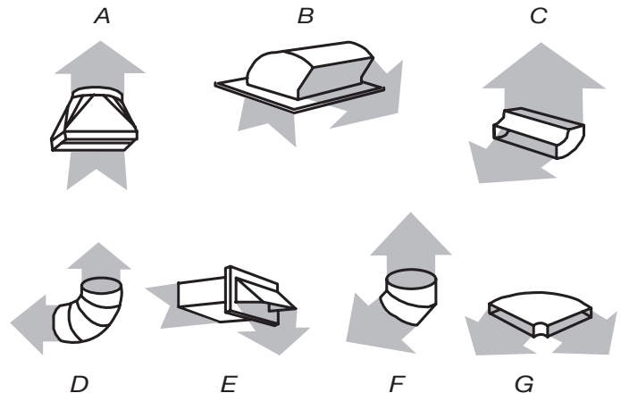
A. Pieza de transición de rectangular a redondo: 3 1/4" x 10" a 6" = 5 pies (83 x 254 mm a 152 mm = 1,5 m) B. Cubierta para el techo: 3 1/4" x 10" = 24 pies (83 x 254 mm = 7,3 m) C. Codo de 90°: 3 1/4" x 10" = 25 pies (83 x 254 mm = 7,6 m) D. Codo de 90°: 6" = 10 pies (152 mm = 3 m) E. Cubierta para la pared: 3 1/4" x 10" = 40 pies (83 x 254 mm = 12,2 m) F. Codo de 45°: 6" = 5 pies (152 mm = 1,5 m) G. Codo plano de 90°: 3 1/4" x 10" = 10 pies (83 x 254 mm = 3 m)
