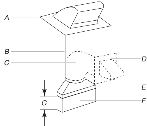
A. Cubierta para el techo B. Ducto de escape redondo con diámetro mínimo de 6" (152 mm) C. Codo (solo para la ventilación a través de la pared) D. Cubierta para la pared E. de transición rectangular a redondo de 3 1/4" x 10" a 6" (83 x 254 mm a 152 mm) F. Pieza para la extensión del ducto de ventilación, al menos 3" (76 mm) de altura G. 3" (7,6 cm)
