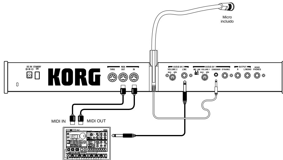
Teclado MIDI, módulo generador de tono, caja de ritmos.
