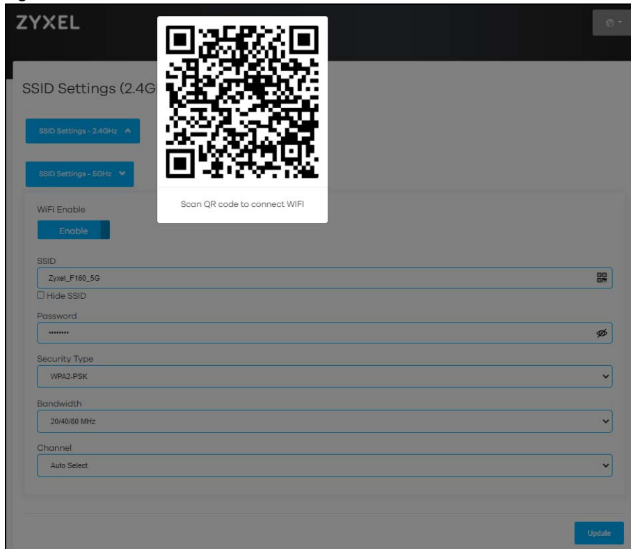
Figure 69 SSID SETTINGS-5 GHz > SSID
