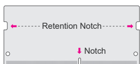
««« DDR4 SO-DIMM
