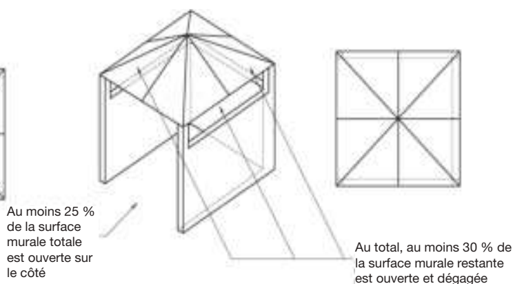
Figure 1d – Exemple d'espace extérieur 4 Espace partiellement fermé doté d'un toit et de plus de deux murs
