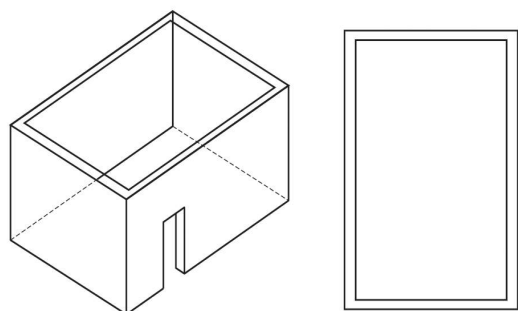
Figure 1a – Exemple d'espace extérieur 1 Murs de tous les côtés, une ouverture permanente
