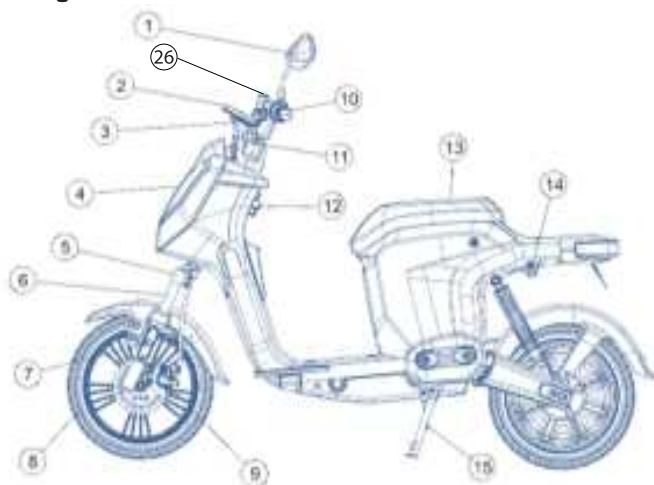
Figura 1. Vista lateral del scooter
