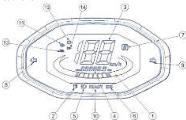
Figura 3. Panell d'instruments (pantalla)
