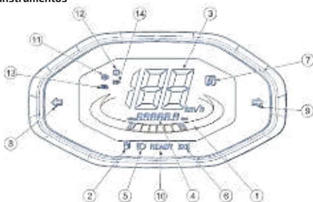
Figura 3. Panel de instrumentos (pantalla)
