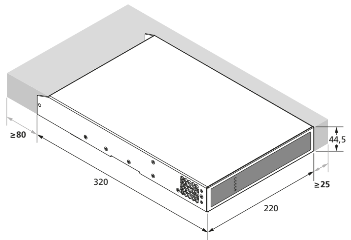
Abb. 4 Belüftungsabstände
