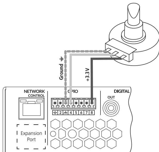
Abb. 5 externer Lautstärkeregler
