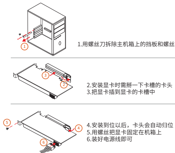
图2-9 显卡安装
