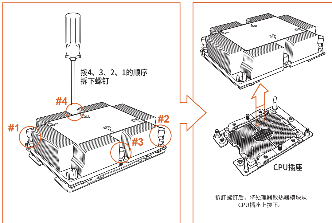
图2-13 CPU拆卸
