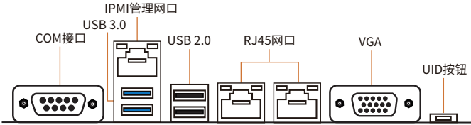
图1-2 整体后置I/O面板展示
