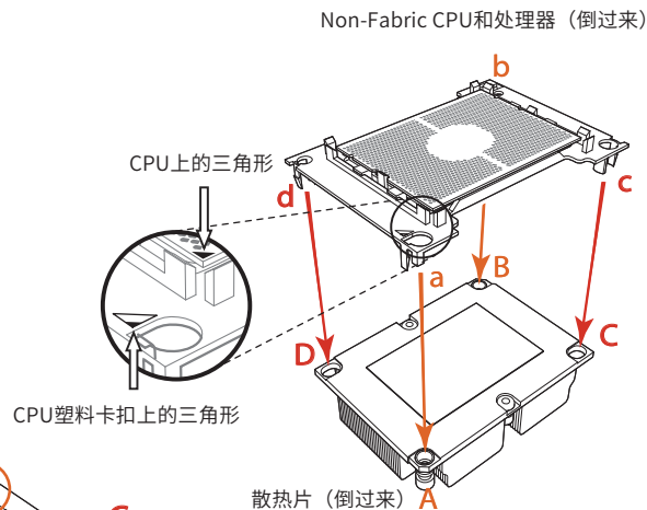
图2-10 CPU安装
