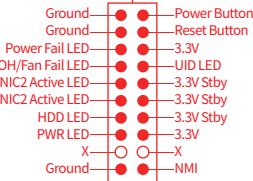
图1-1 X11D-16D双路主板图解
