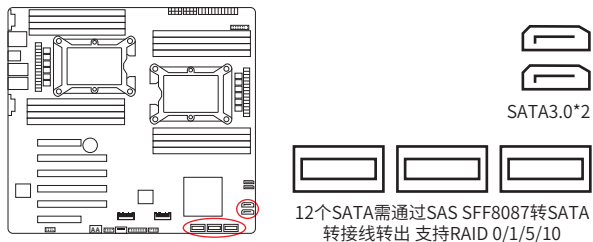
图2-6 SATA接口
