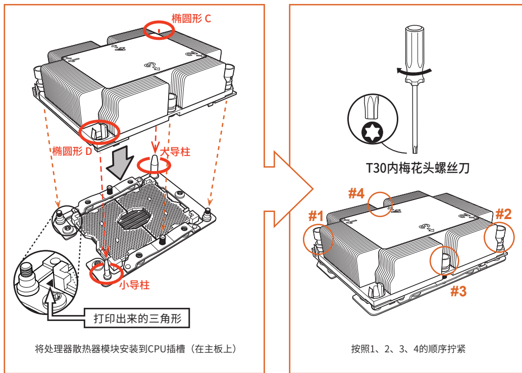
图2-12 CPU安装
