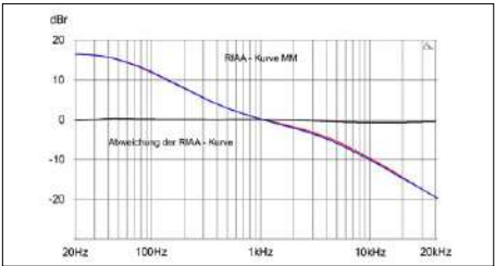
Auch der Phono-Pre ist offensichtlich keine Alibi-Funktion, die RIAA-Kurve ist sehr ordentlich.
