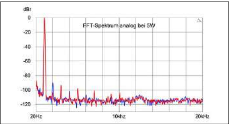
Das FFT-Spektrum des Denon sieht exzellent aus, von Rauschen und Verzerrungen keine Spur.
