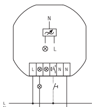
Aansluitvoorbeeld
