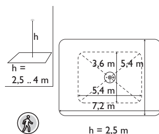
Detectiebereikdiagram
