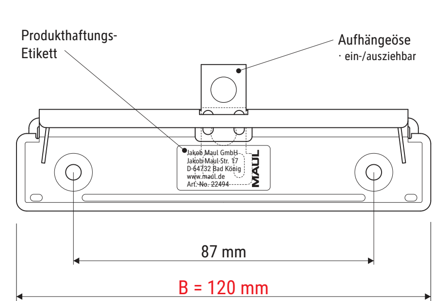
Rückseite
