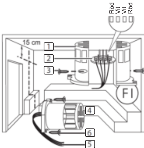
Bild 5 Montering av urogivare
