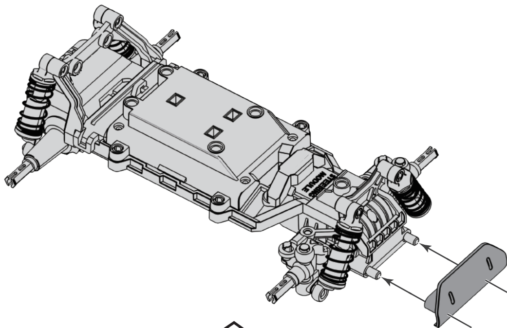
Stoßfänger / Bumper F2-1 1x
