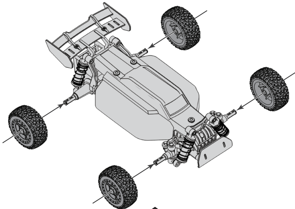
Räder / Wheels 4x
