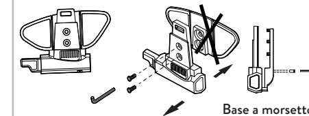
Base a morsetto
