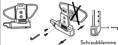
Schraubklemme
