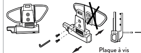
Plaque à vis
