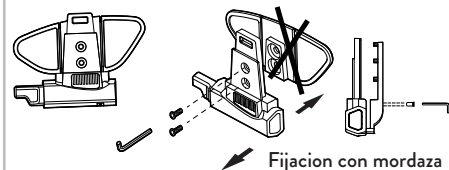
Fijación con mordaza
