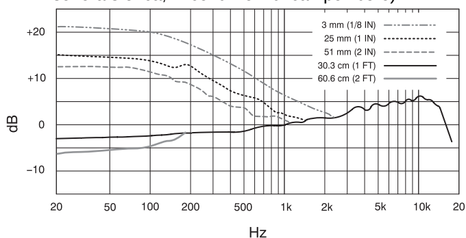
RISPOSTA IN FREQUENZA TIPICA FIGURA 2
