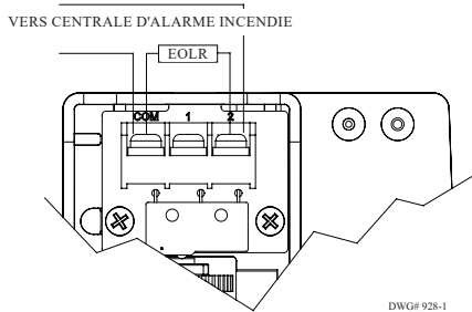
Raccordement du signal basse pression Fig. 4
