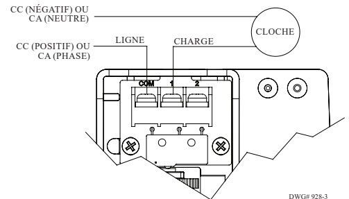
Raccordement d'une alarme sonore locale de débit Fig. 6
