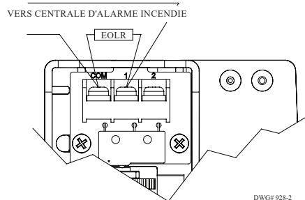
Raccordement du signal de débit Fig. 5
