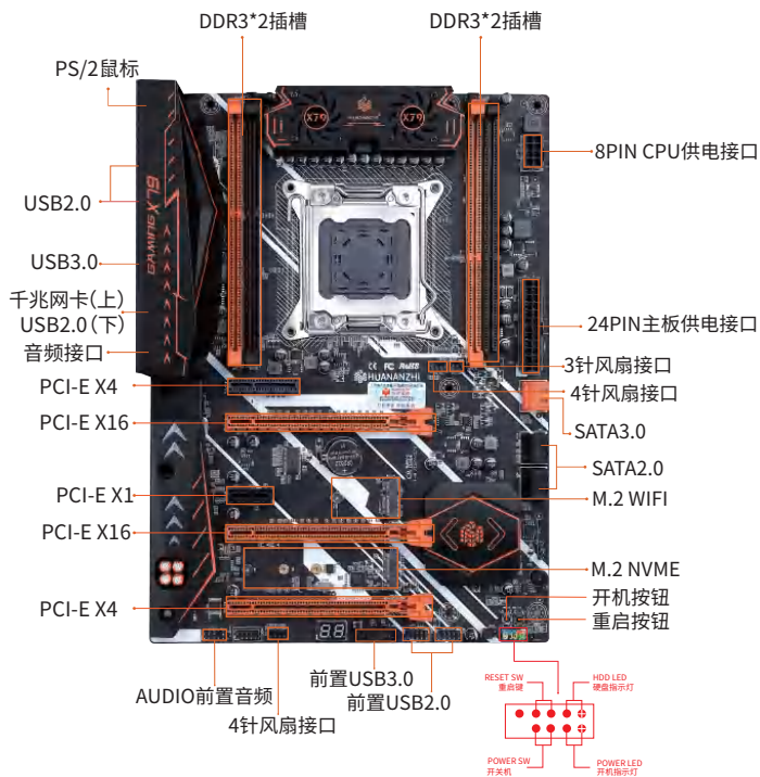
图1-1 X79至尊V7.1主板图解
