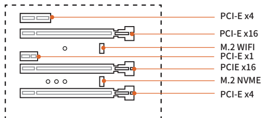
图2-4 PCI扩展插槽
