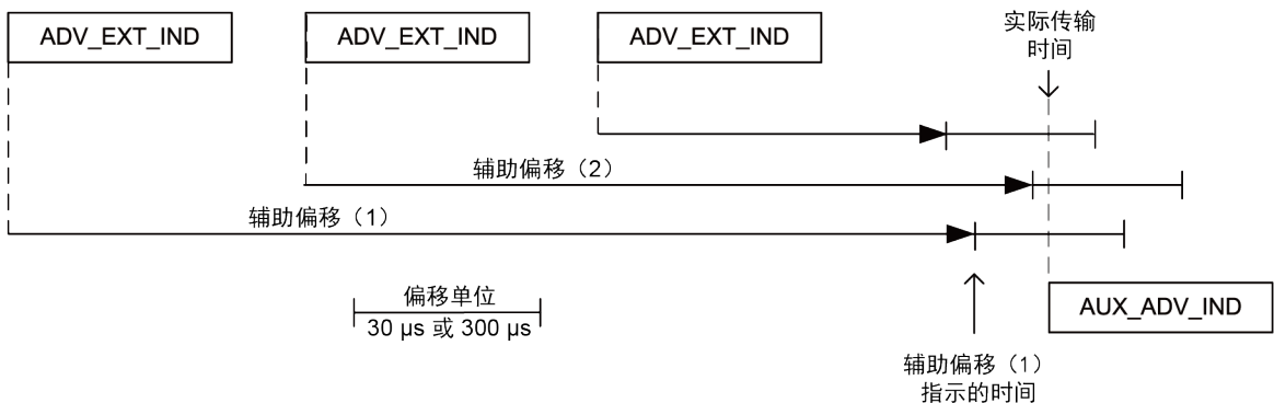
图 19. 广播组示例
