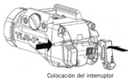
Colocación del interruptor
