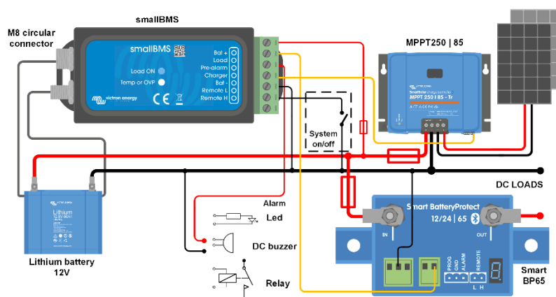
Figure 1 : exemple d'application pour un système CC hors réseau avec un interrupteur d'allumage/arrêt entre L et le pôle négatif de la batterie.
